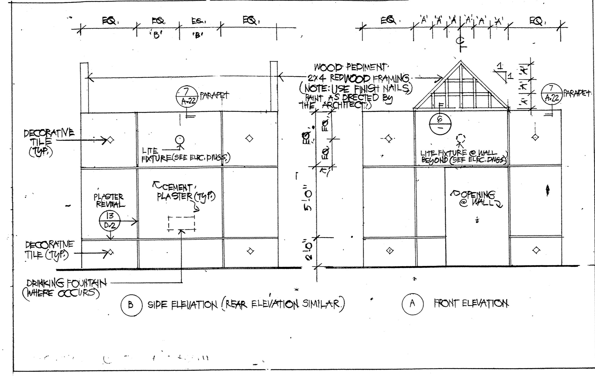
TOILET ROOM 1/4"=1'-0"
