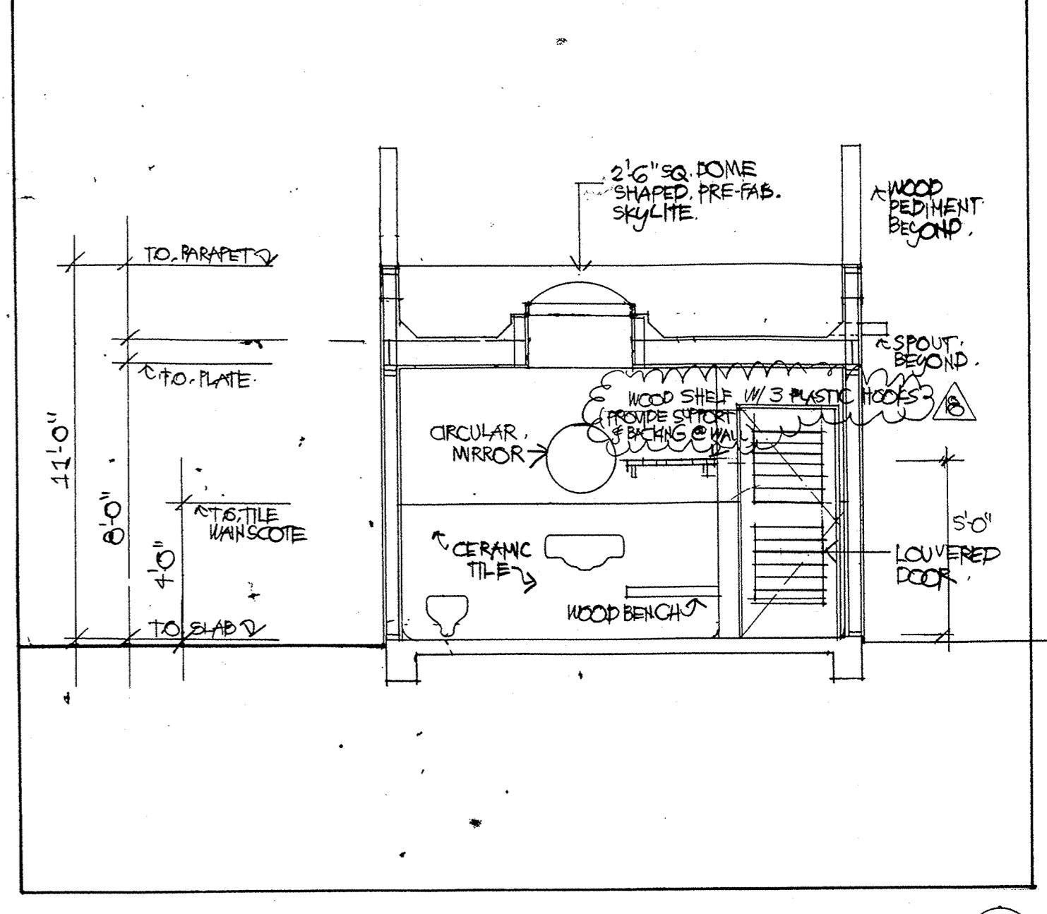
TOILET ROOM 1/4"=1'-0"
