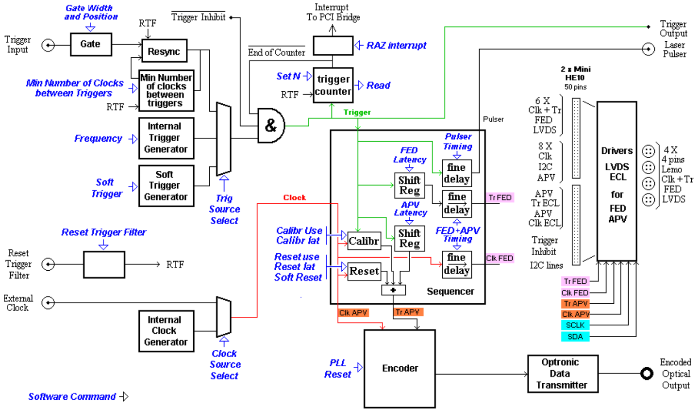
Figure 6. Fonctionnal block diagram
