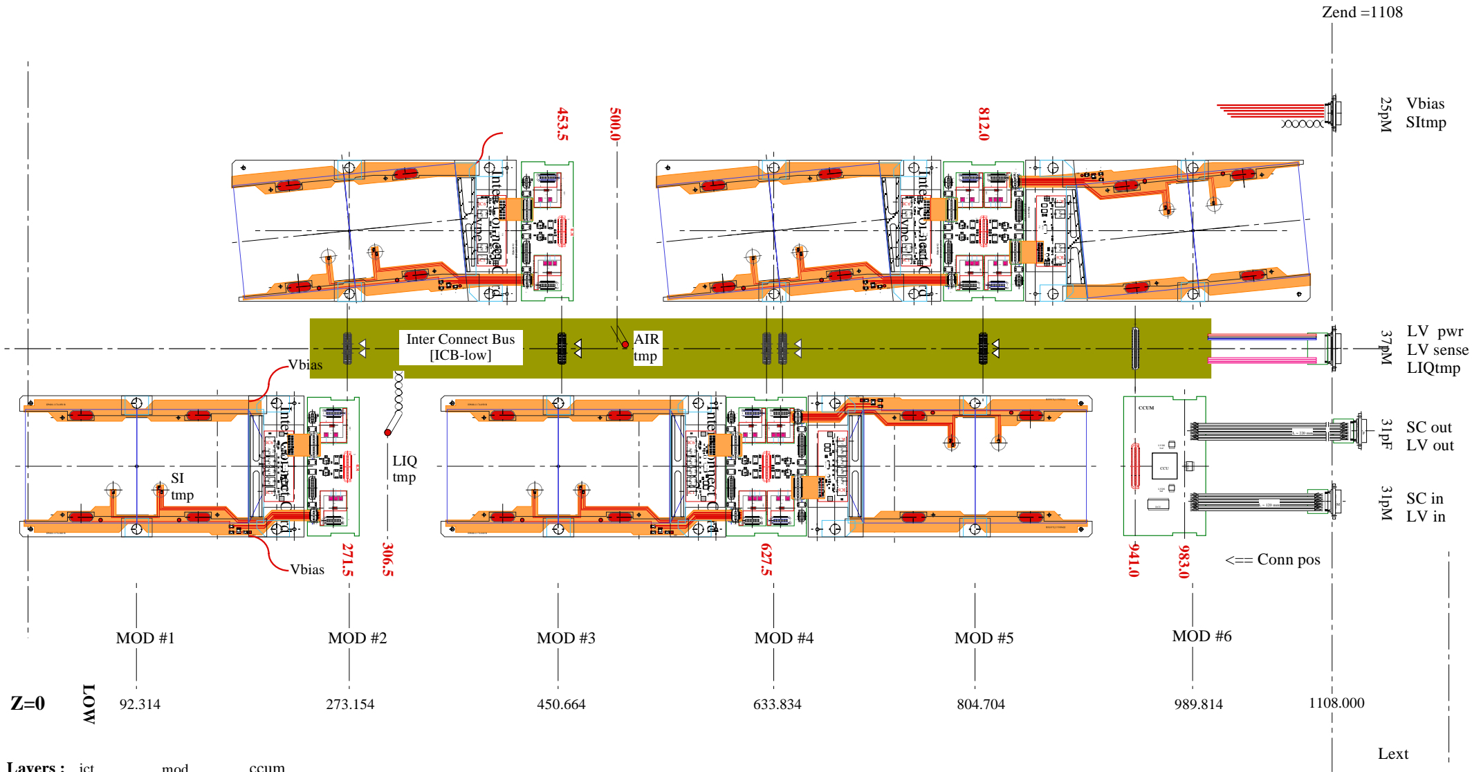
TOB, layer 1 and 2, DS Ladders
